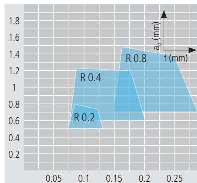
Optимальное стружколомение
