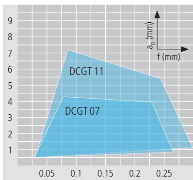
Оптимальное стружколание
