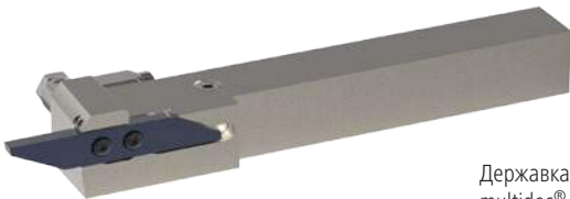
Державка «AK» со встроенной подачей охлаждающей жидкости для revolverных станков
