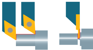
Исполнение «TWIN» с внутренним охлаждением
