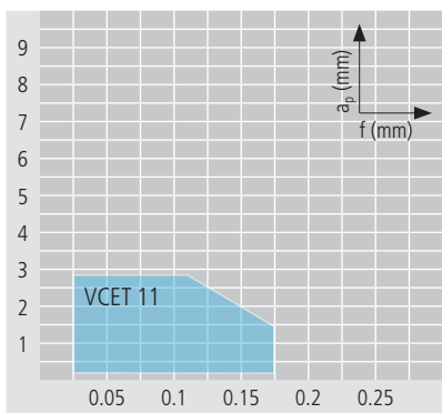
Оптимальное стружколомание
