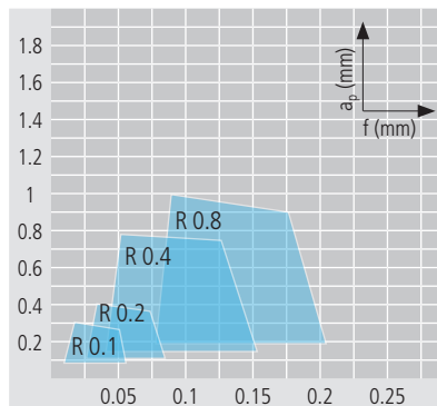
Optимальное стружколомение
