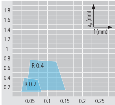
Optимальное стружколомание
