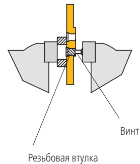
Выпрессовывание
