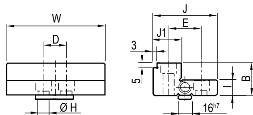
Art. 814 Base mobile per ganasce fisse - Movable base for fixed jaws
