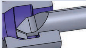
Schneideinsätze Rückwärtsdrehen
